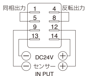
【端子配列】
